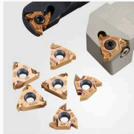
Roscado
